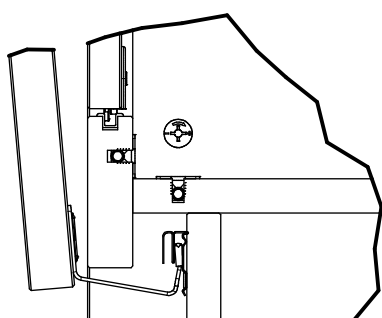
AH ( 1 : 4 )
